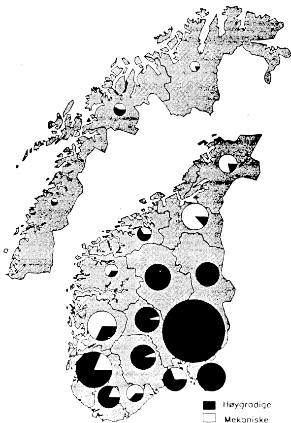
Figur 2. Avløpsrenseanlegg. Hydraulisk kapasitet (P.E.) fordelt på mekaniske og høygradige avløpsrenseanlegg. Fylke. 1991.
